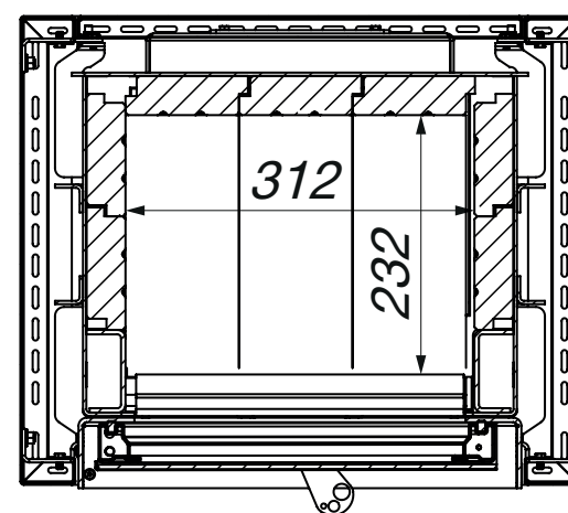
B-B (1 : 10)
